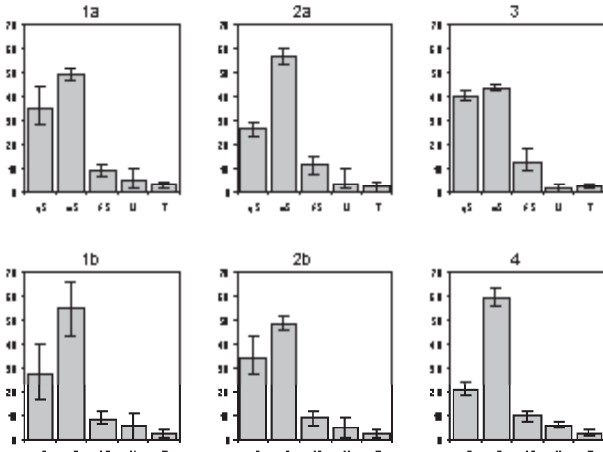
Abb. 1: Korngrößenverteilung innerhalb der sechs Profile. Angegeben sind die Mittel-, Maximal- und Minimalwerte in Gew. %
